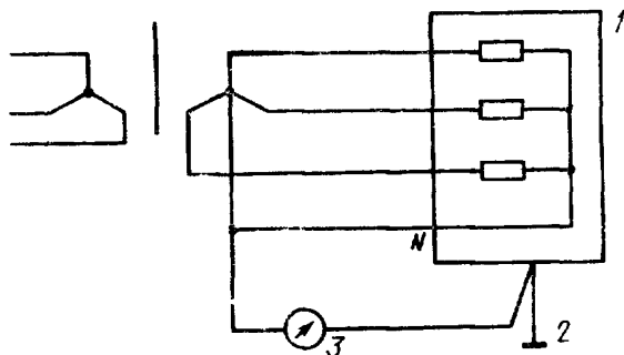
1 — испытуемое устройство; 2 — соединительный зажим заземления; 3 — измерительный прибор
