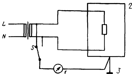
1 — измерительный прибор; 2 — испытуемое устройство; 3 — соединительный зажим заземления
