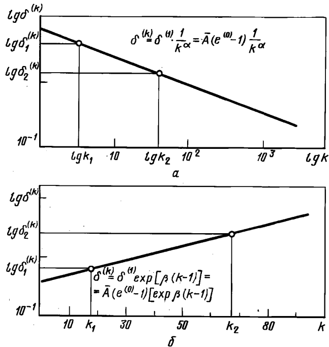
а — циклическое упрочнение; б — циклическое разупрочнение
