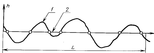
1 — реальный профиль; 2 — средняя прямая
