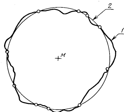
1 — реальный профиль; 2 — средняя окружность
