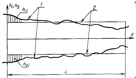
1 — реальный профиль; 2 — средний профиль продольного сечения
