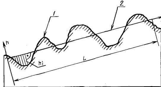
1 — реальный профиль; 2 — средняя прямая
