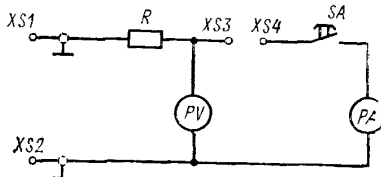
РА—амперметр; PV—вольтметр.
