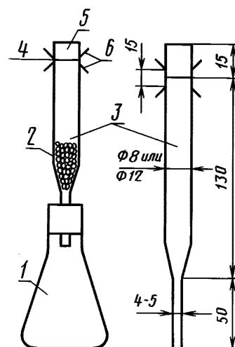
Прибор для определения мышьяка визуальнометрическим методом
