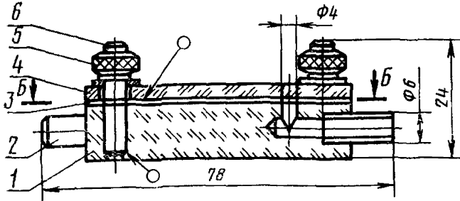
Камера счетная проточная
