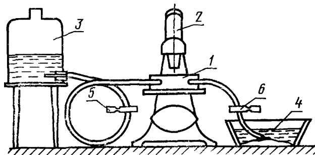
1—счетная камера; 2—микроскоп; 3—склянка; 4—емкость; 5, 6—зажимы
