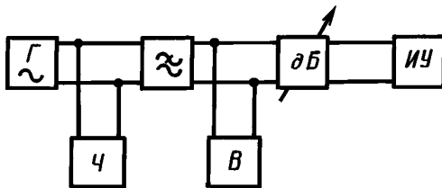
Г — измерительный генератор; \approx — фильтр нижних частот; дБ — магазин затуханий; Ч — частотомер; В — образцовый измерительный прибор; ИУ — измеритель уровня
