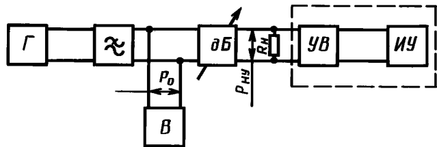
Г — измерительный генератор; \approx — фильтр нижних частот; В — образцовый измерительный прибор; дБ — магазин затуханий; УВ — выносное устройство; ИУ — измеритель уровня; R_{н} — нагрузка магазина затуханий
