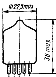
Расположение штырьков РШ-8— по ГОСТ 7842—71
