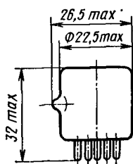
Расположение штырьков РШ-8 по ГОСТ 7842—71
