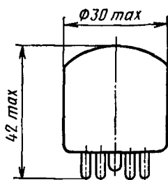
Расположение штырьков РШ-24— по ГОСТ 7842—71
