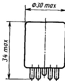
Расположение штырьков РШ-24 по ГОСТ 7842—71
