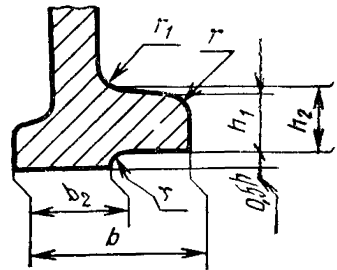
Вариант исполнения бурта по разъему опок для ручной и пескометной формовки
