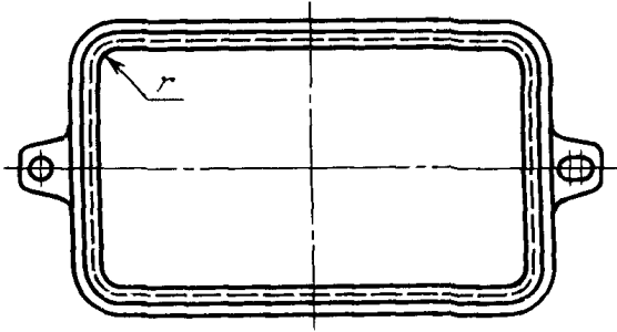
Радиусы сопряжения стенок опок
