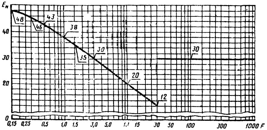
E_n — напряженность поля радиопомех, дБ; F — частота, МГц
