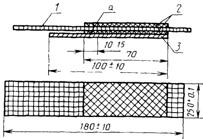
Схема образца
