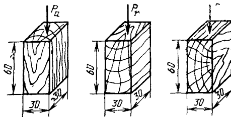
a — ( P_a ) — нагрузка, сжимающая образец вдоль волокон, b — ( P_r ) — нагрузка, сжимающая образец поперек волокон в радиальном направлении, в — ( P_t ) — нагрузка, сжимающая образец поперек волокон в тангентальном направлении
