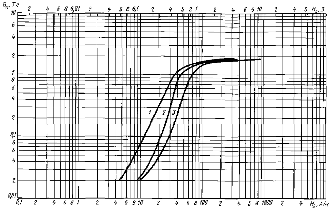
Кривые намагничивания стали марки 3424 (Э360А) для частот: 1 — 400 Гц, 2 — 1000 Гц, 3 — 3000 Гц
