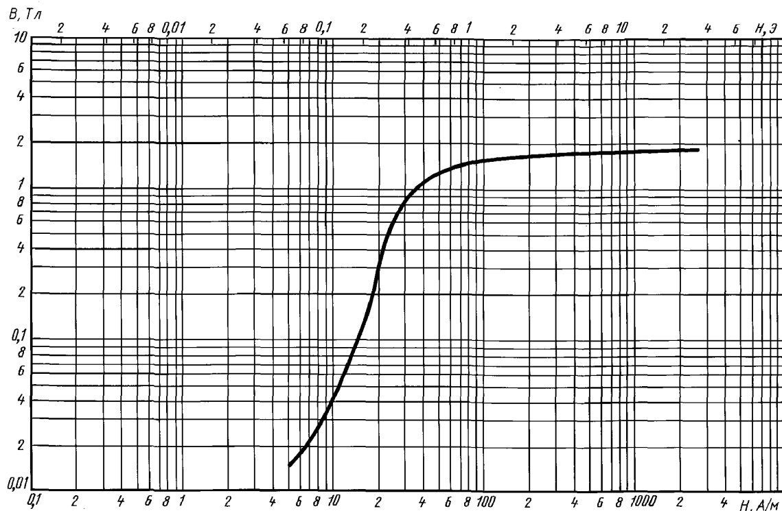
Кривые намагничивания стали марки 3424 (Э360А)
