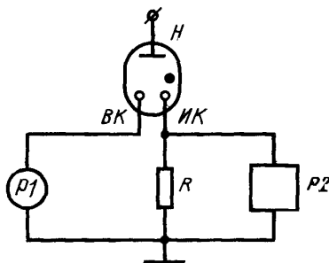
R — измерительный резистор; P1 — измеритель постоянного тока; P2 — осциллограф или импульсный вольтметр; H — испытываемый индикатор; BK — вспомогательный катод; IK — индикаторный катод
