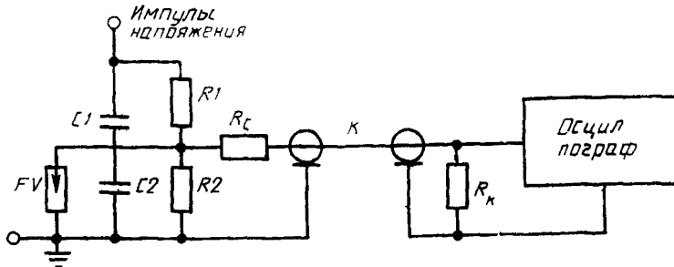
FV — разрядник; K — коаксиальный кабель; R1, R2 — сопротивления высоковольтной и низковольтной частей делителя соответственно; C1, C2 — емкости высоковольтной и низковольтной частей делителя соответственно; R c — согласующее сопротивление; R к — волновое сопротивление кабеля
