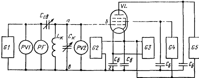
G1 —генератор напряжения; PVI , PV2 —вольтметры переменного тока; PF —измеритель частоты; Cсв —конденсатор связи; Lк —катушка индуктивности контура; Cк —конденсатор контура; G2 , G3 , G4 , G5 —источники питания; VL —испытуемая лампа; Cб —блокировочный конденсатор
