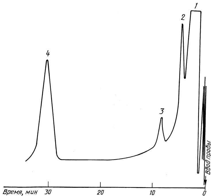
1 — 1,2-дихлорэтан; 2 — 1,1,2-трихлорэтан; 3 — додекан; 4 — 1,1,2,2-тетрахлорэтан
