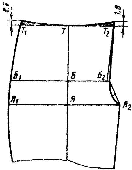
Черт. 3
