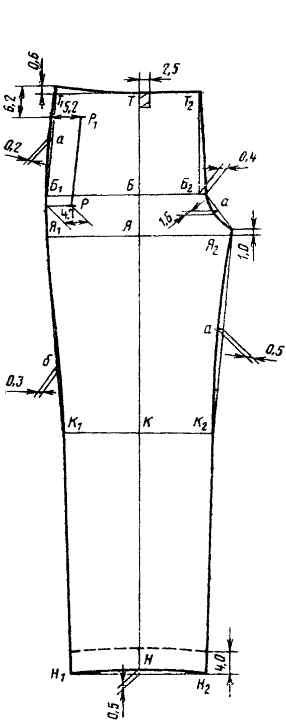
Черт. 1
