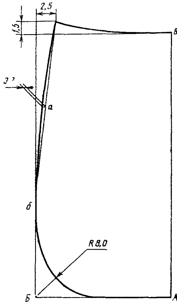
Черт. 11
