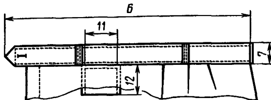
Черт. 4
