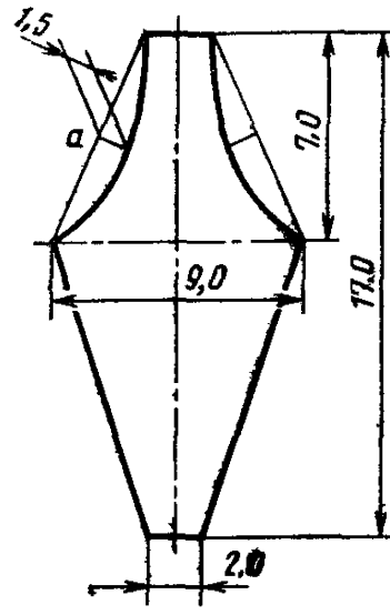
Черт. 10
