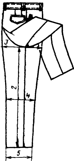
Черт. 2
