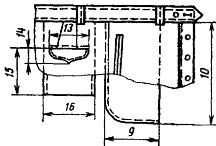
Черт. 5
