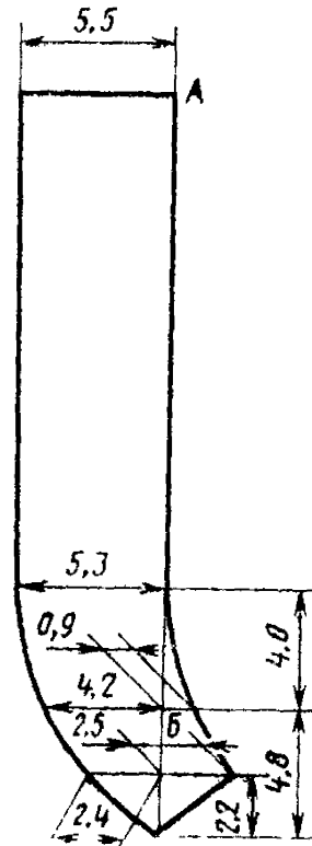
Черт. 5
