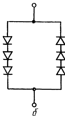
Черт. 8
