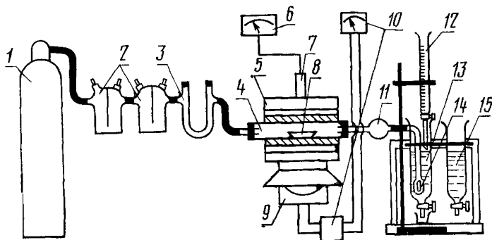
1 — кислородный баллон 2 — промывные склянки 3 — U-образная трубка, 4 — фарфоровая трубка, 5 — трубчатая печь, 6 — гальванометр, 7 — термопара, 8 — фарфоровая лодочка, 9 — терморегулятор, 10 — автотрансформатор с амперметром, 11 — стеклянный шарик, 12 — микробюретка, 13 — поглотительный сосуд, 14 — барботер, 15 — сосуд с раствором сравнения
