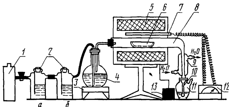
1 — баллон с азотом 2 — промывные склянки 3 — элекгропитка 4 — парообразователь 5 — трубка пасты 6 — кварцевая лодочка 7 — термометр 8 — кварцевая трубка 9 — холодильник 10 — отводная трубка с барботером 11 — колода приемник 12 — микровысмер 13 — автотрансформатор
