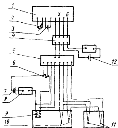
1—потенциометр, 2—гальванометр; 3, 7, 12—батареи, 4—инверсионный переключатель; 5—двухполюсный многоточечный переключатель; 6—образцовая катушка сопротивления; 8—магазин сопротивлений; 9—образцовый термометр сопротивления; 10, 11—термопары.
