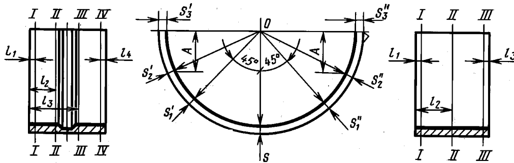
Вкладыши с кольцевой масляной канавкой
