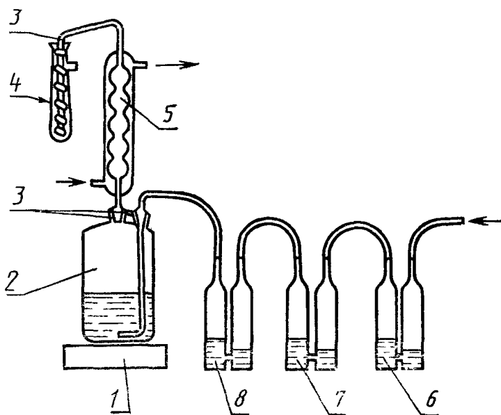
1 — электроплитка, 2 — реакционный сосуд с восстановительной смесью, 3 — шлифы, 4 — приемник с щелочным раствором гидросиламина и ЭДТА (спиральная кварцевая насадка, приваренная к наружной стороне выходной трубки обратного холодильника), 5 — обратный холодильник, 6—7 — барботеры с раствором пирогаллола 250 г/дм 3 в растворе едкого калия 250 г/дм 3 , 8 — барботер с дистиллированной водой
