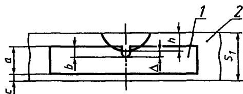
1 — образец; 2 — составная пластина
