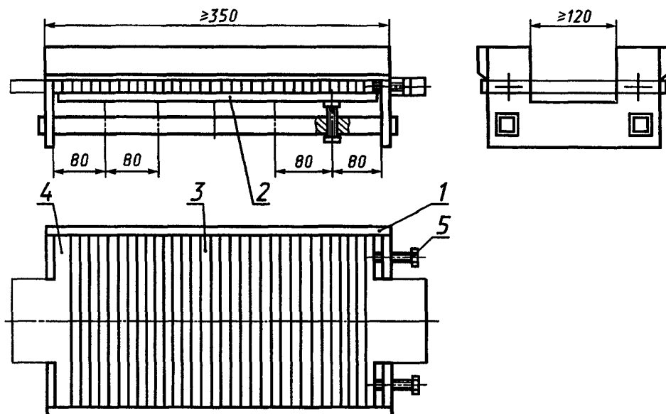
1 — планка опорная; 2 — планка прижимная; 3 — пластина составная; 4 — планка приставная; 5 — болт для стягивания брусков в горизонтальной плоскости
