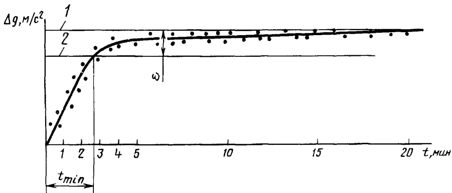
Определение длительности переходного процесса
