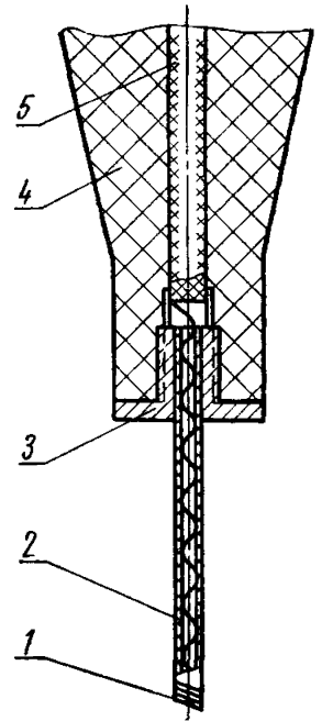
1 — катушка - датчик; 2—трубка; 3—втулка; 4—ручка; 5—кабель 75-омный со штыревым разъемом.
