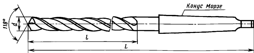
Вариант исполнения сверл с шейкой
