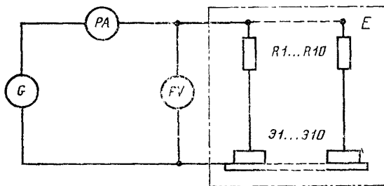
R1 \dots R10 —резисторы; \mathcal{E}1 \dots \mathcal{E}10 —электроды
