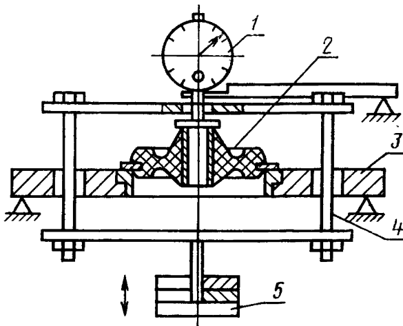
1—индикатор; 2—амортизатор; 3—опорная поверхность; 4—загрузочная рамка; 5—груз.
