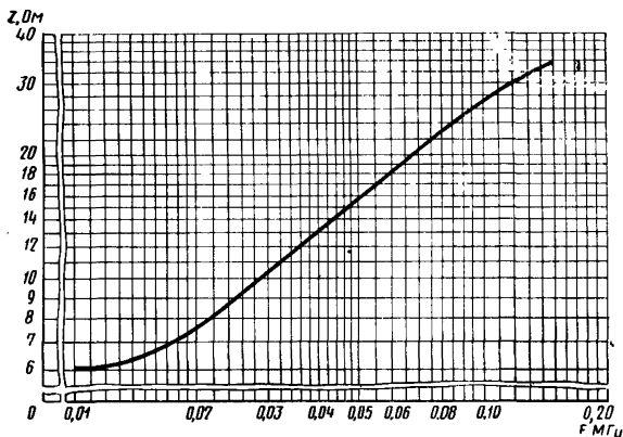
Модуль входного полного сопротивления V-образного эквивалента сети типа I
