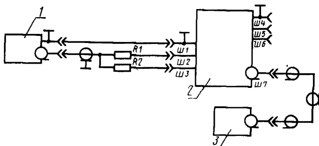
1 — генератор синусоидальных сигналов; 2 — эквивалент сети; 3 — измеритель радиопомех; R_1=R_2=150 \pm 1,5 Ом; Ш1, Ш4 — разъемы «ЗЕМЛЯ»; Ш2, Ш3 — разъемы «ИСТОЧНИК РАДИОПОМЕХ»; Ш5, Ш6 — разъемы «СЕТЬ ЭЛЕКТРОПИТАНИЯ»; Ш7 — разъем «ИЗМЕРИТЕЛЬ РАДИОПОМЕХ»
