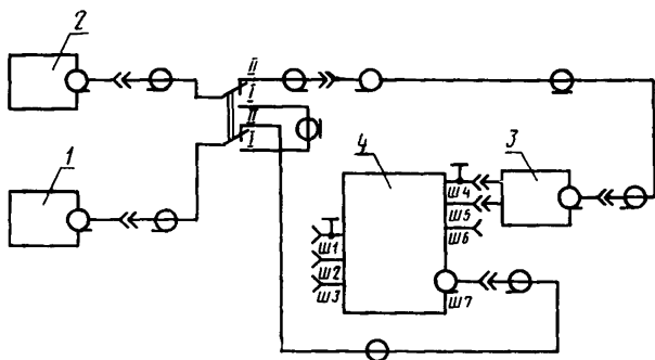
Схема проверки затухания фильтра эквивалента сети
