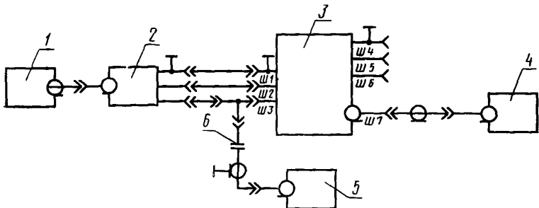
Схема проверки сетевого коэффициента помехозащищенности измерителя радиопомех
