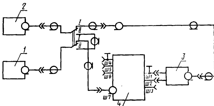
Схема проверки переходного затухания V-образного эквивалента сети
