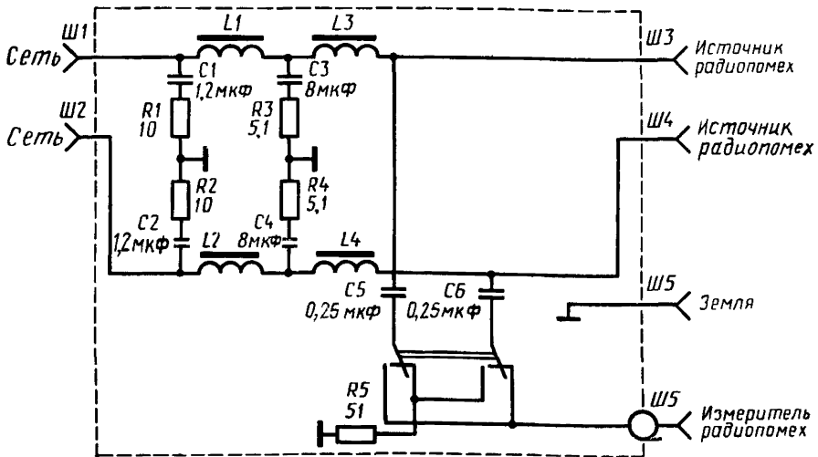
Схема электрическая принципиальная двухфазного V-образного эквивалента сети типа 1
