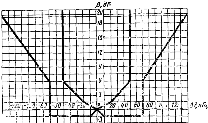
\beta — значение характеристики избирательности; \Delta f — расстройка
