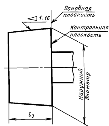
Калибр-пробка К-Г
