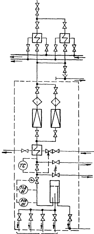
К анализатору черт. 2
