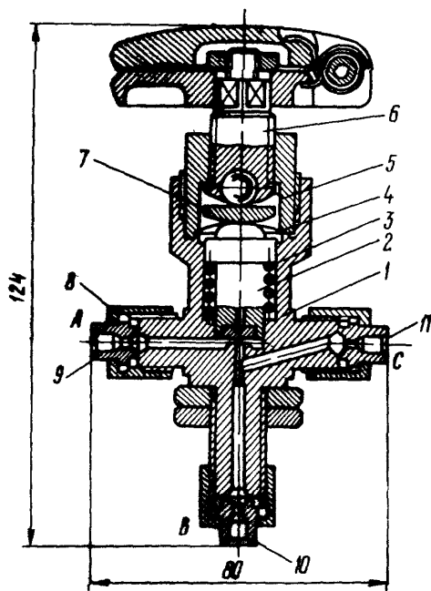
Рис.4. Вентиль трехходовый кислородный ВВ-2МС: 1 - корпус; 2 - клапан; 3 - пружина; 4 - мембрана; 5 - крышка; 6 - шпиндель; 7 - сухарь; 8 - гайка накидная; 9, 10, 11 - шпидели
