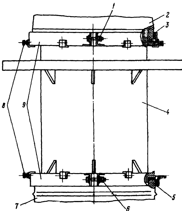
Рис.12. Узел крепления крышек вводов 220 кВ: 1,6 - болт М12х130-58; гайка М12,5, шайба 12-005; 2 - верхняя фарфоровая крышка; 3,5 - прокладка резиновая; 4 - соединительная втулка; 7 - нижняя фарфоровая крышка; 8 - болт М12х40-58, гайка М12,5; 9 - подукорытце
