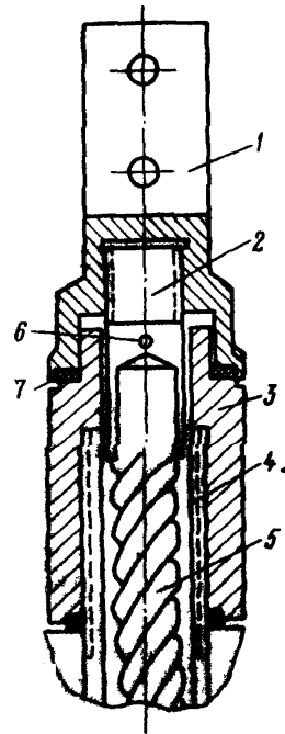
Рис.17. Контактное соединение ввода МТУ-110/600;
