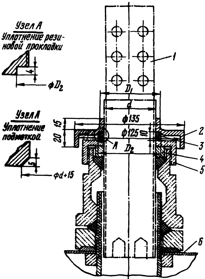
Рис. II. Реконструкция уплотнения верхнего узла вводов трансформаторов;
