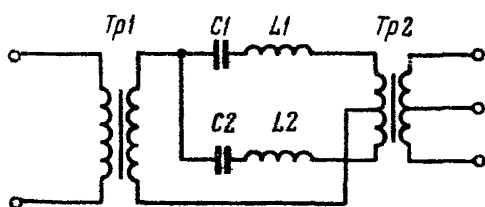
Рис. 20. Схема линейного фильтра передатчика
