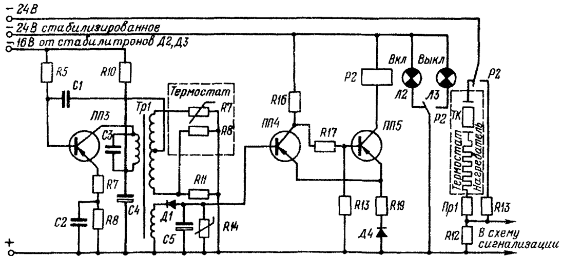
Рис. 24. Схема регулирования температуры в термостате
