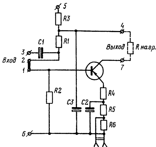
Рис. 26. Типовая схема модуля
