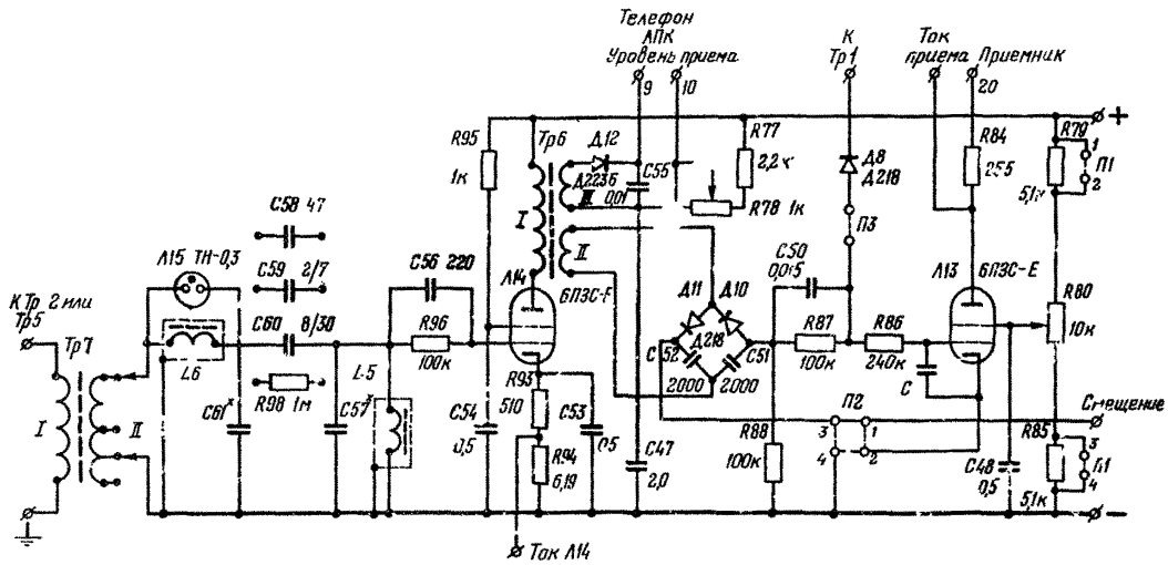
Рис.7. Схема приемника (элементы схемы включены для работы с дифференциально-фазной защитой при одночастотной настройке)
