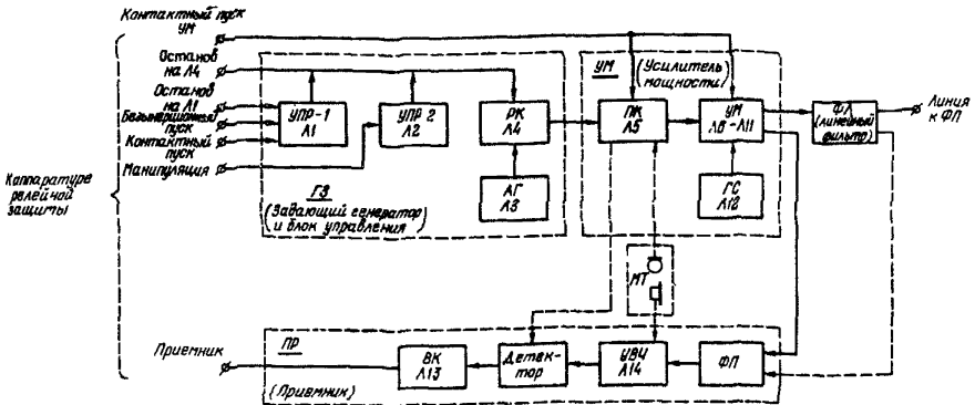
Рис.1. Структурная схема приемопередатчика УЗР-70
