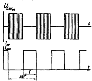
Рис. 9. Форма манипулированных ВЧ сигналов на выходе передатчика и соответствующие им импульсы тока приемника
