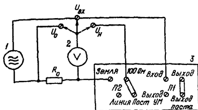
Рис.23. Схема для измерения затухания передачи ФЛ:
