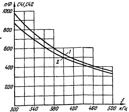
Рис.40. Зависимость значения емкости контуров ФЛ от заданной частоты настройки (диапазон частот 301-500 кГц; L3 = L4 = 0,3 \text{ мГ} ):
