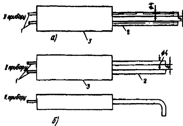
Рис. 1. Эскиз зонда:
