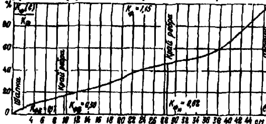
Рис. 17. График для определения коэффициента форм изолятора НС-2 (чертеж И-324) и коэффициентов формы
