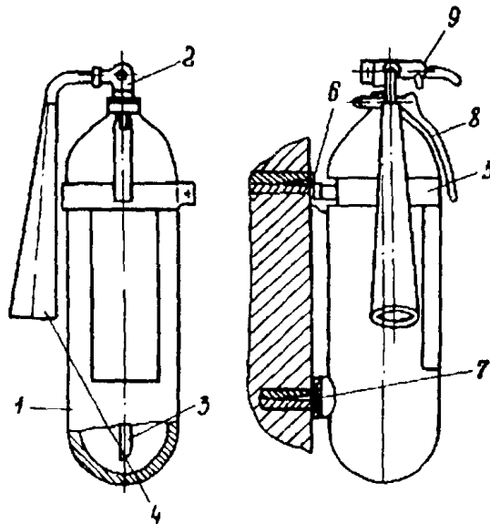
Рис. 7. Ручной углекислотный огнетушитель ОУ-5 (ОУ-8):
