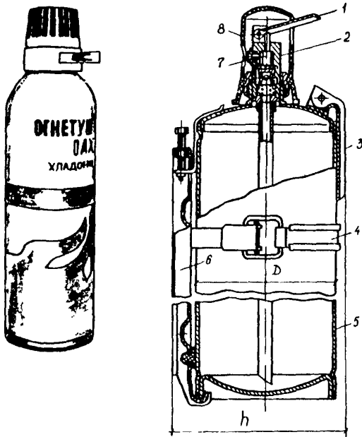
Рис. 11. Хладоновый огнетушитель ОУБ-3А (ОУБ-7А):
