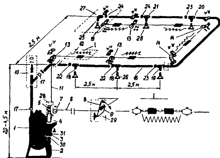
Рис. 14. Схема устройства стационарного автоматического огнетушителя ОПА:
