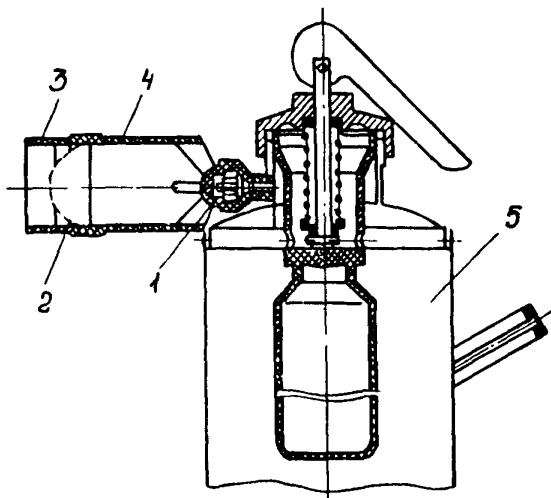
Рис. 2. Пенный насадок:
