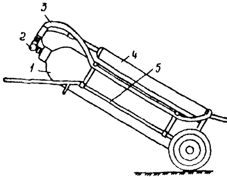
Рис. 8. Передвижной углекислотный огнетушитель ОУ-25:
