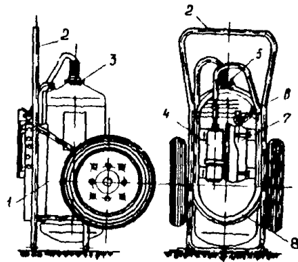
Рис. 4. Передвижной воздушно-пенный огнетушитель ОВП-100:
