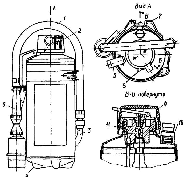
Рис. 3. Ручной воздушно-пенный огнетушитель ОВП-10:
