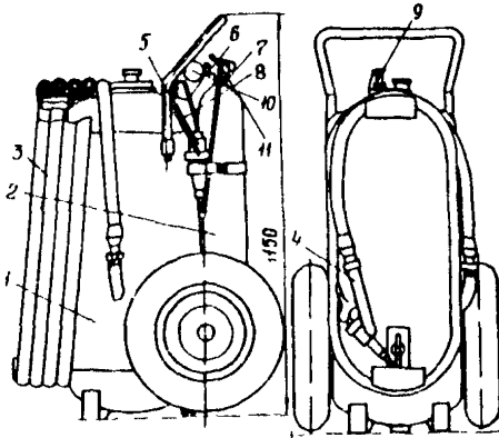
Рис. 13. Общий вид передвижного порошкового огнетушителя ОП-100:
