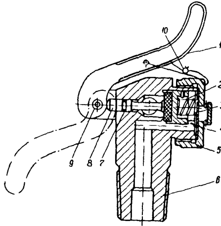
Рис. 10. Запорно-пусковое устройство рычажного типа УН-52:
