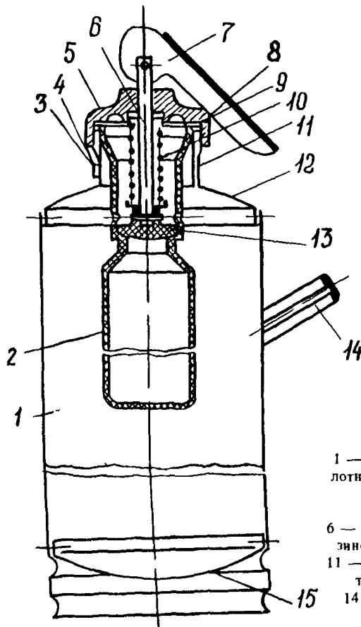
Рис. 1. Огнетушитель ОХП-10:
