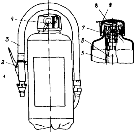
Рис. 12. Общий вид ручного порошкового огнетушителя ОП-5:
