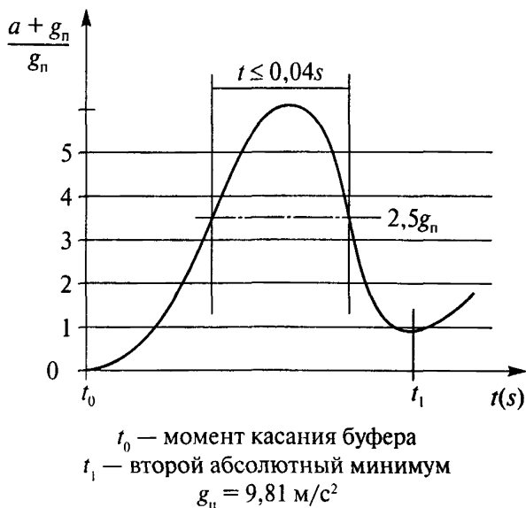
Рис. 1. График торможения
