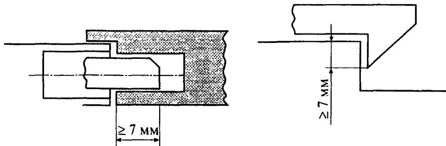
Рис. 5. Запирающее устройство автоматического замка двери шахты
