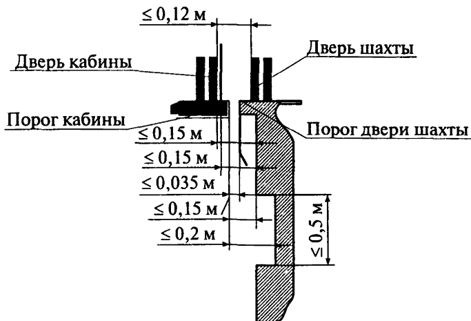
Рис. 3. Расстояния между элементами кабины и шахты
