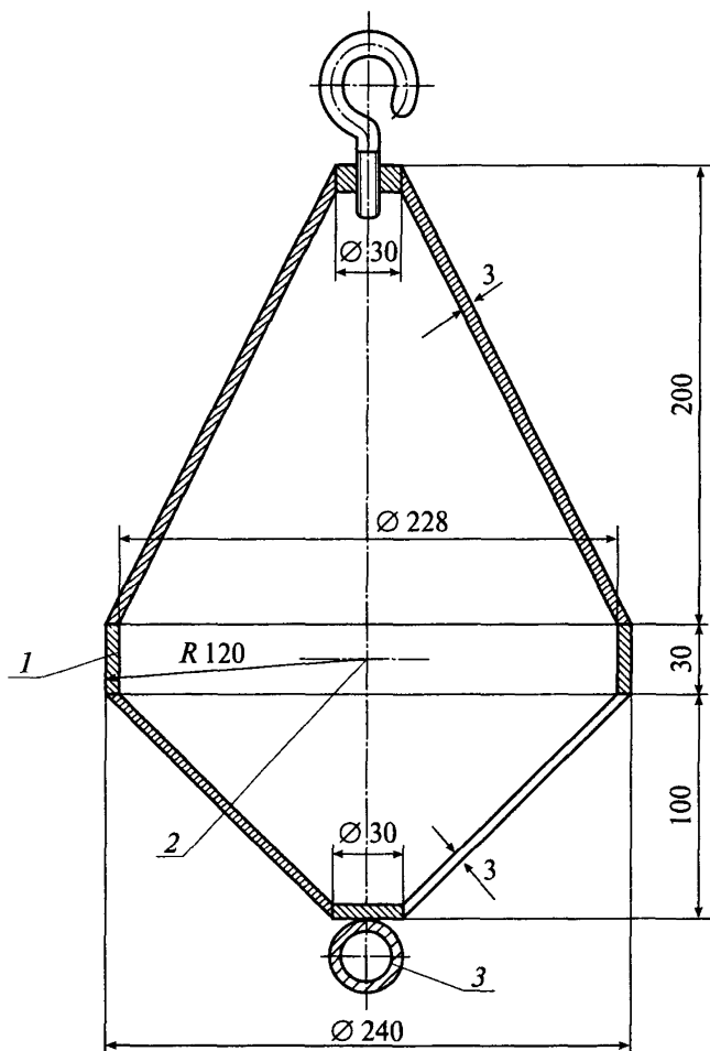
Рис. 1. Маятник для жесткого удара:
