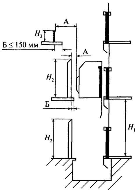
Рис. 1. Расстояние до движущихся элементов лифта:
