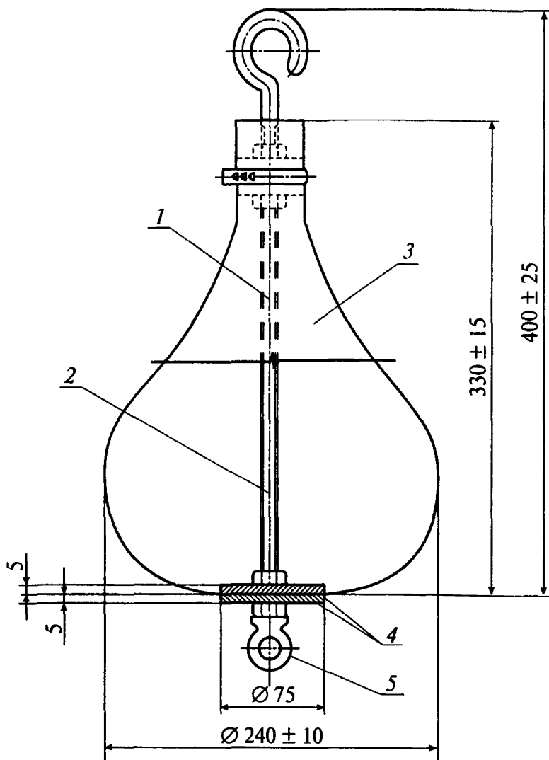
Рис. 2. Маятник для нежесткого удара:
