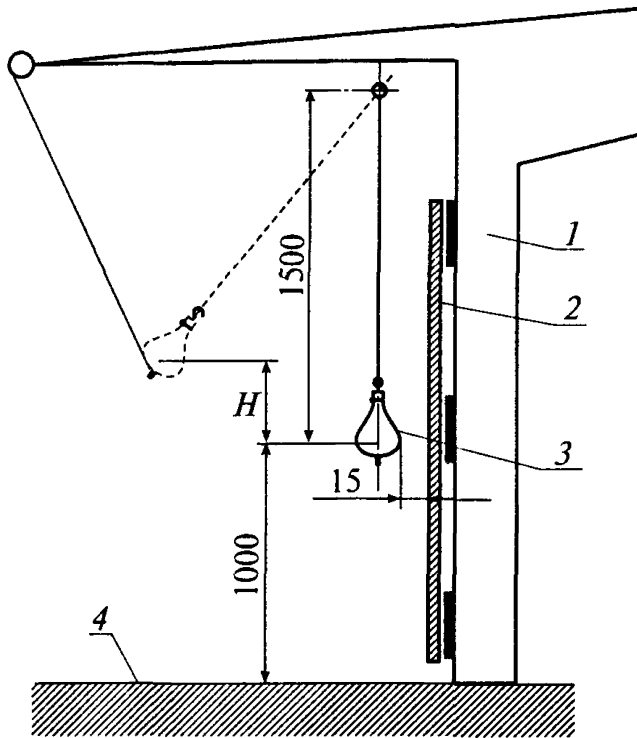
Рис. 3. Высота падения на испытательном стенде: 1 — рама; 2 — испытываемая стеклянная панель; 3 — маятник; 4 — уровень пола, относящийся к испытываемой стеклянной панели; H — высота падения
