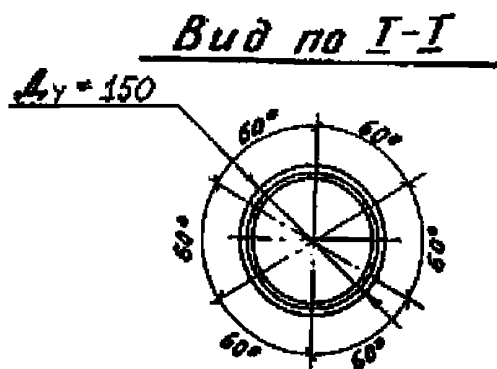
Рис. 13. Труба гофрированная из полиэтилена низкого давления с водопримными отверстиями заводского изготовления
