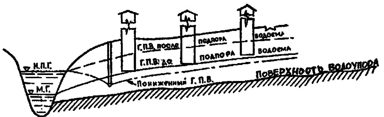
Рис.6. Схема берегового дренажа
