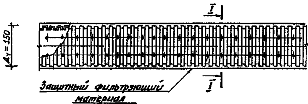
Рис. 12. Труба поливинилхлоридная с водопрёмными отверстиями и с заделкой стыков
