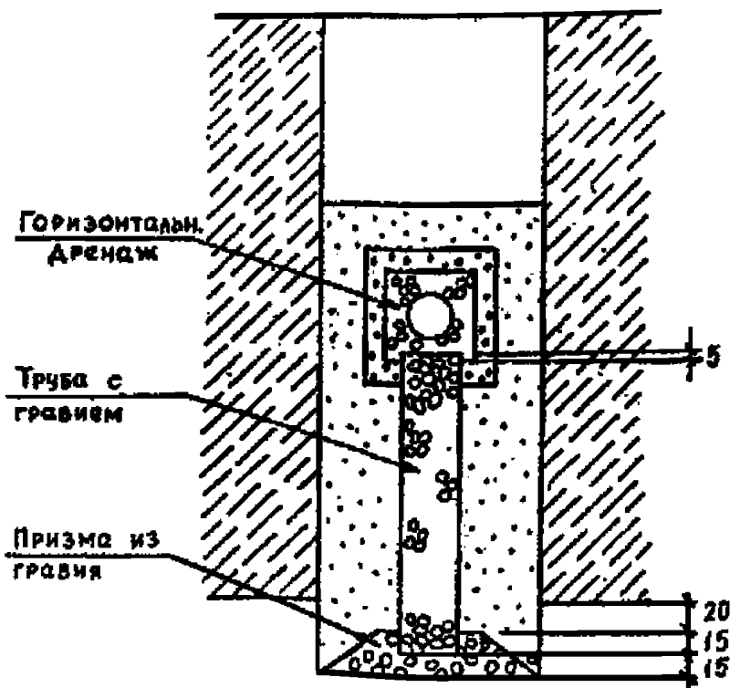
Рис.5. Комбинированный дренаж с вертикальным самоизливающимся колодцем
