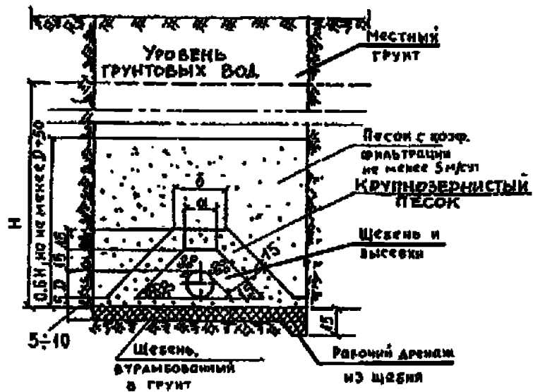
Рис.1. Дренаж совершенного типа
