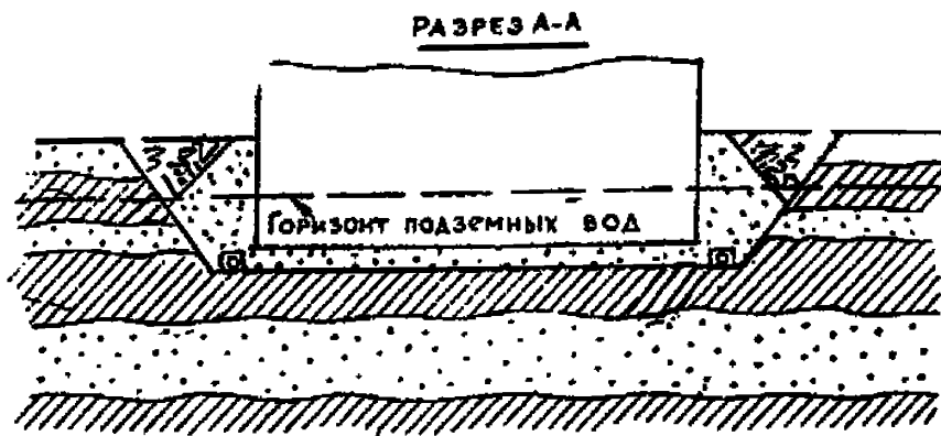
Рис.8. Схема кольцевого дренажа
