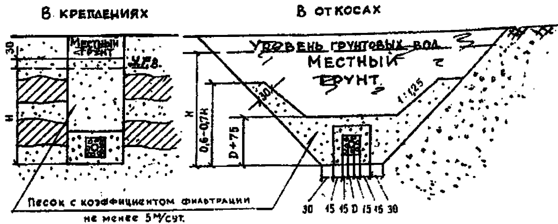
Рис.4. Схемы засыпки граншей с фильтрующей призмой дренажа несовершенного типа
