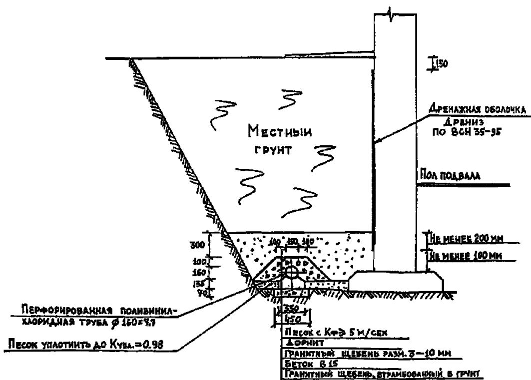
Рис. 14. Пристенный дренаж с применением поливинилхлоридных труб на бетонном основании и дренажной оболочкой "Дрениз"
