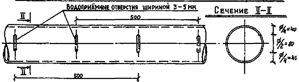
Рис. 12. Труба поливинилхлоридная с водопрёмными отверстиями и с заделкой стыков
