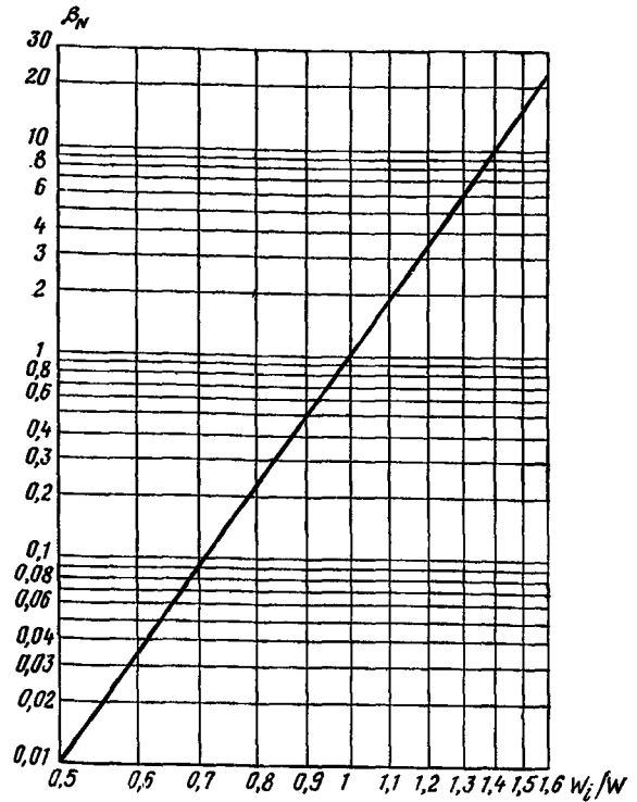
Рис. 19. График для определения коэффициента \beta_N
