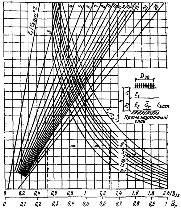
Рис. 24. Номограмма для определения удельных растягивающих напряжений при изгибе \bar{\sigma} в промежуточном слое из материала, обработанного органическими или неорганическими вяжущими
