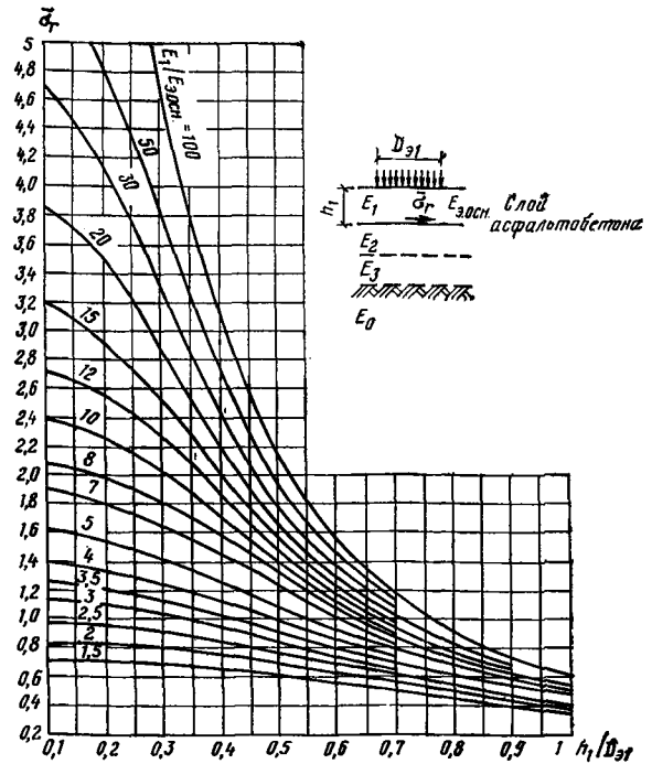
Рис. 23. Номограмма для определения удельных растягивающих напряжений при изгибе \bar{\sigma} в асфальтобетоне
