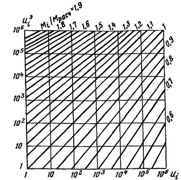
Рис. 18. Номограмма для определения эквивалентного числа приложений нагрузки u_i^3
