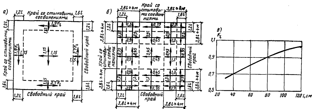
Рис. 14. Значения переходных коэффициентов K
