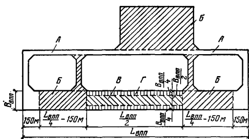
Рис. 2. Схема деления покрытий аэродрома на группы участков
