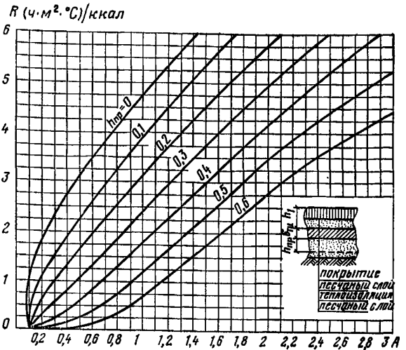
Рис. 11. Номограмма для определения термического сопротивления теплоизоляции R
