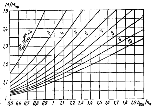
Рис. 25. График для определения соотношения толщин искусственного основания h_{осн} из материалов, обработанных вяжущими, и бетонного или армобетонного покрытия h_{п}
