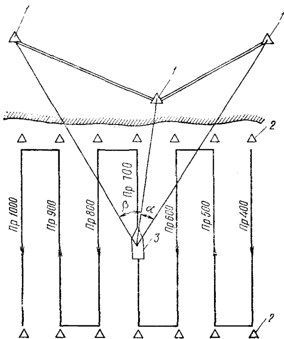
Черт. 9. Промер по заданному направлению с определением координат глубин обратной засечкой:
