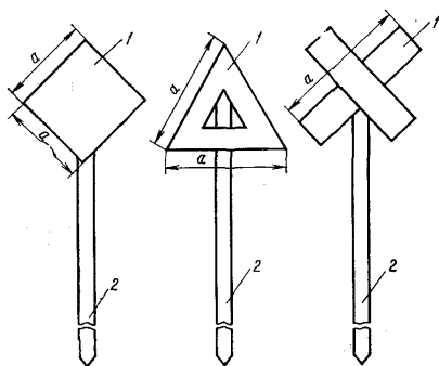
Черт. 25. Типы вешек для обозначения границ участка дноуглубительных работ: 1 — топовая фигура вешки; 2 — шест вешки; a — размер топовой фигуры
