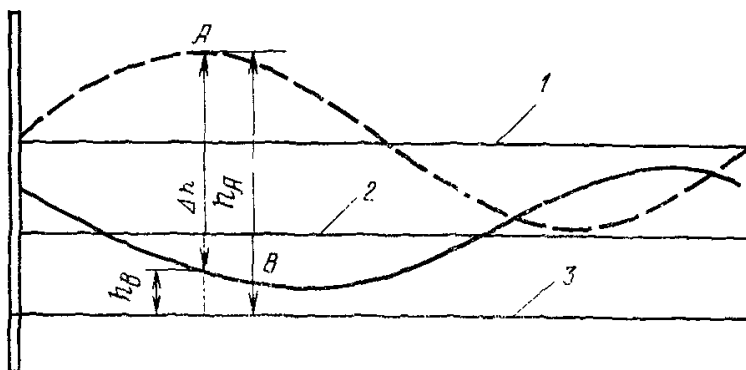
Черт. 27. Совмещенный график колебаний уровня моря на уровнечных постах A и B : 1 — средний уровень поста A ; 2 — средний уровень поста B ; 3 — нуль глубин; h_B - h_A высоты мгновенного уровня моря над нулем глубин, м
