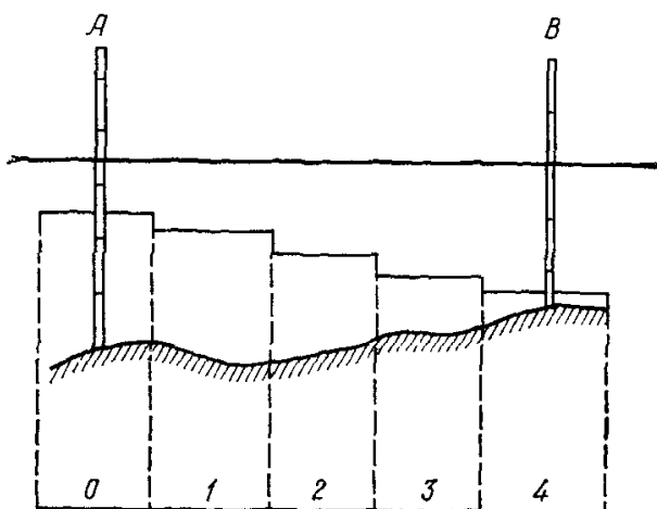
Черт. 28. Разбивка зон: 0, 1, 2, ..., 4 — номера зон; A и B — уровнечные посты
