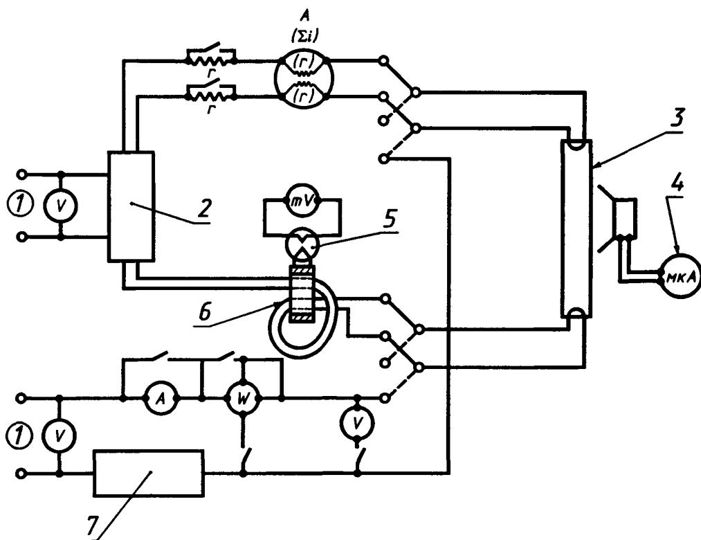
1 — источник питания; 2 — испытуемый ПРА; 3 — трансформатор тока; 4 — термопара; 5 — номинальная лампа; 6 — фотоэлемент; 7 — образцовый ПРА
