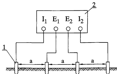
1 – стальные электроды; 2 – измерительный прибор
