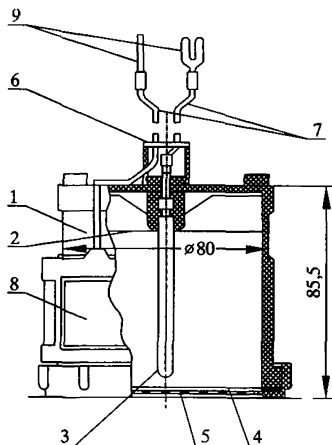
Стационарный медносульфатный электрод сравнения типа ЭСН-МС или ЭНЭС-1
