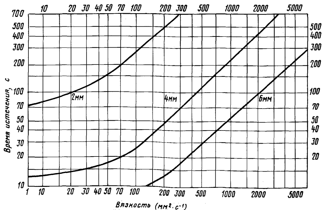
Зависимость времени истечения ( \tau ) от вязкости ( \text{мм}^2/\text{с} ) лакокрасочного материала в вискозиметрах с различным диаметром сопла
