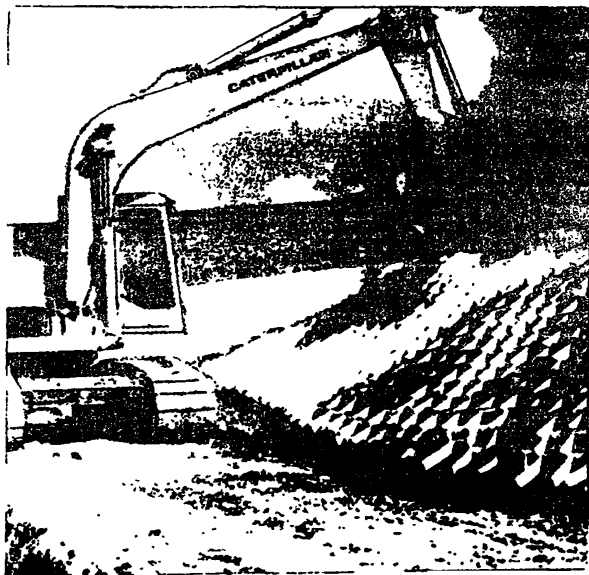
Рис.19. Засыпка георешеток типа Armatex растительным грунтом.
