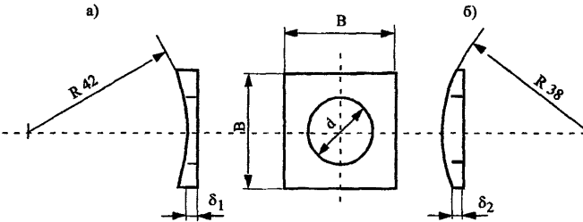
Рис. 1. Шайбы для болтов (размеры в мм): а – плосковогнутые; б – плосковыпуклые; d – диаметр отверстия в шайбе (согласно ГОСТ 11371-68*); B – размер квадратной шайбы, принимаемый равным наружному диаметру стандартной круглой шайбы (согласно ГОСТ 11371-78*); \delta_1 – не менее 3; \delta_2 – не менее 2
