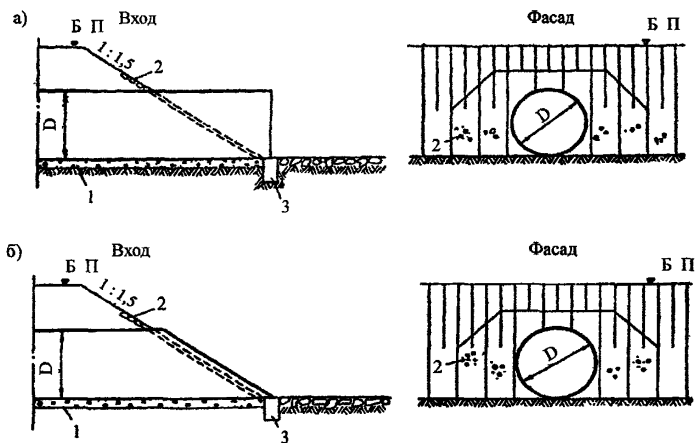
Рис. 1. Схема конструкции трубы верхней стороны насыпи: 1 – подушка основания; 2 – укрепление откоса; 3 – противофильтрационный экран
