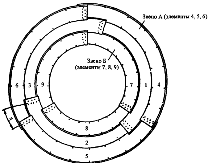
Рис. 5. Сборка секции трубы из звеньев ( d = 1,5 м, вид с торца): цифрами показан порядок установки элементов; а – сдвижка (забег) продольных стыков
