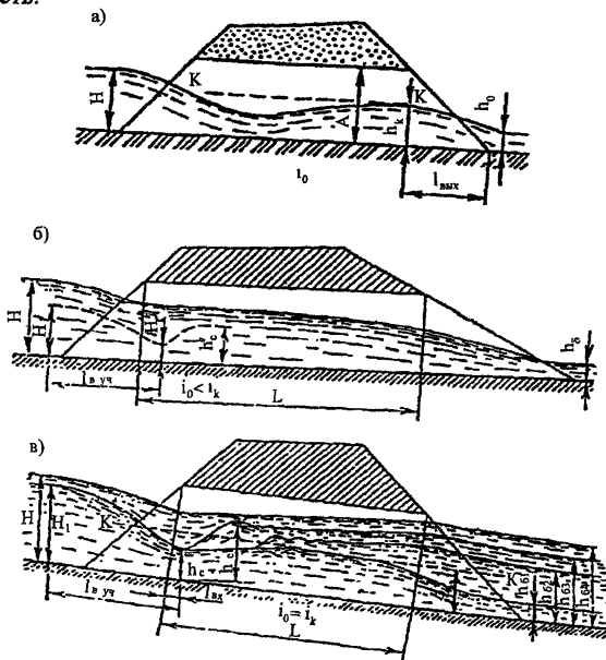
Рис. 1. Схема протекания воды в равнинной трубе при безнапорном режиме: а – «короткая»; б – «длинная»; в – «незатопленная» ( h_{62} , h_{63} ) и «затопленная» с нижнего бьефа ( h_6 )
