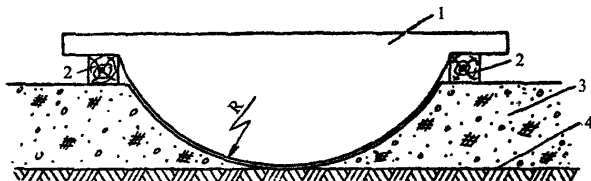
Рис. 4. Вырезка грунтового ложа по шаблону: 1 – шаблон; 2 – подкладка из брусьев; 3 – нулевой слой; 4 – верх подушки
