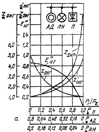
Зависимость параметров комплексной нагрузки Z_{1НГ} , Z_{2НГ} , Z_{0НГ} , E_{НГ} от ее состава
