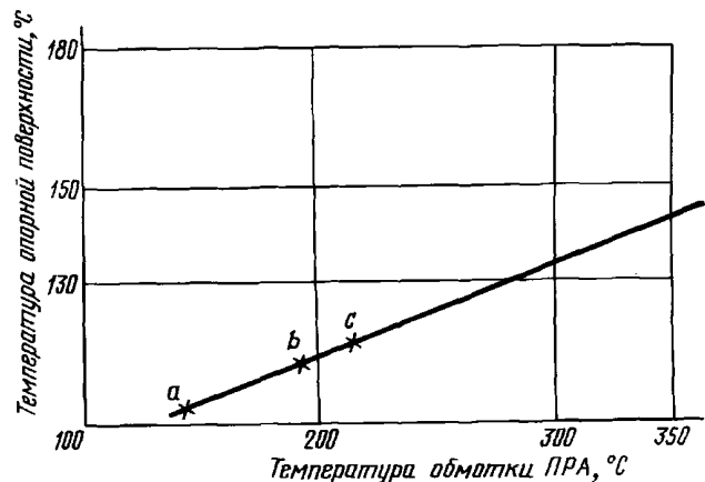
a, b, c — измеренные значения температуры при 0,9-; 1,0 и 1,1-кратном номинальном напряжении
