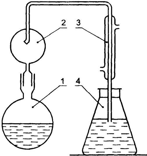
1 — круглодонная колба, 2 — каплеуловитель, 3 — холодильник, 4 — приемная колба
